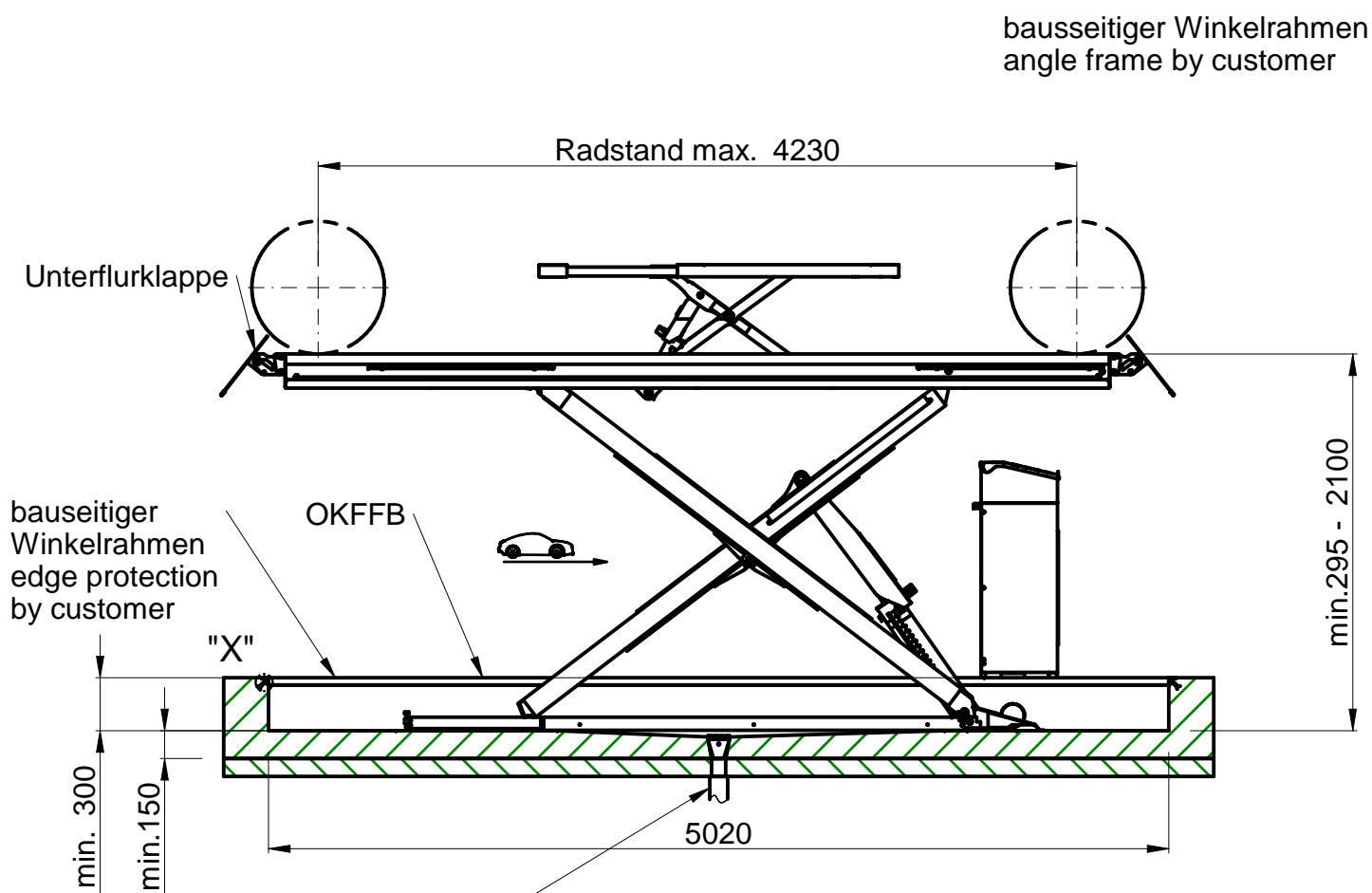
DETTAGLIO "X" 1:5
